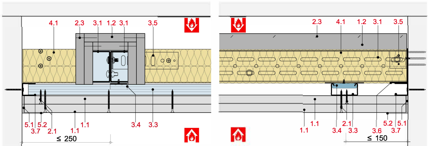
Querschnitt
