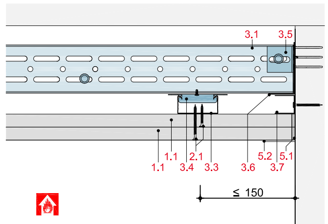
Längsschnitt
