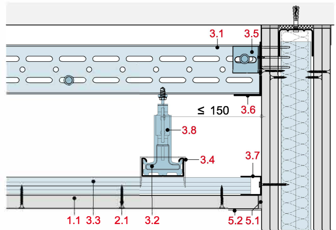
Querschnitt
