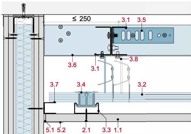
Längsschnitt
