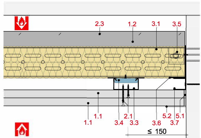
Längsschnitt
