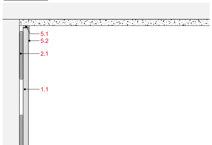
Deckenanschluss an Massivdecke
