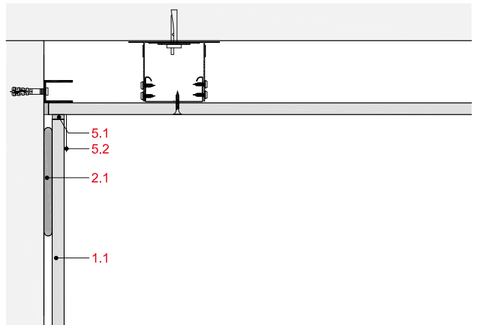
Deckenanschluss an Deckenbekleidung
