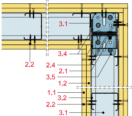
Schnitt C-C
