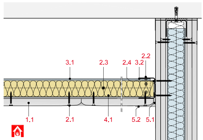
FD21 D WT 30 2 Längsschnitt
