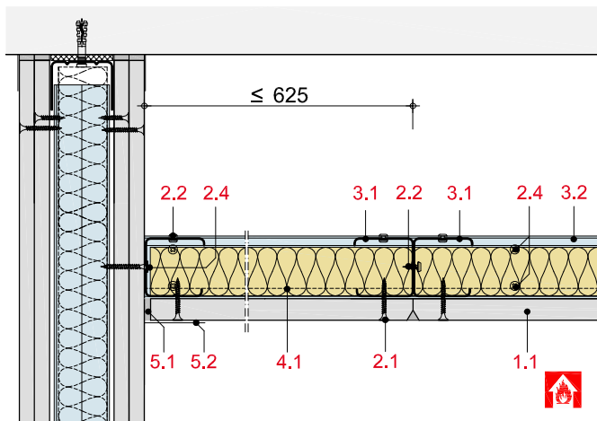
FD21 D WT 30 1 Querschnitt
