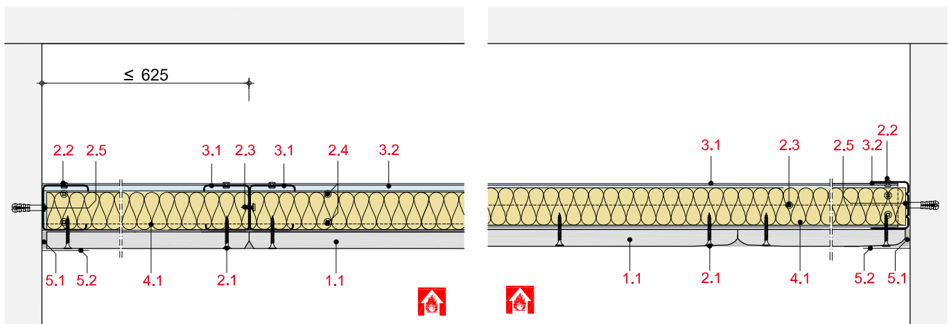
FD21 D WM 30 1 Querschnitt
