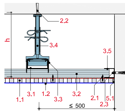
Schnitt B
