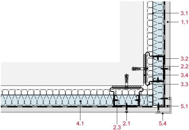
Ausbildung einer Außenecke, Vorsatzschale mit Rigips Deckenprofil CD
