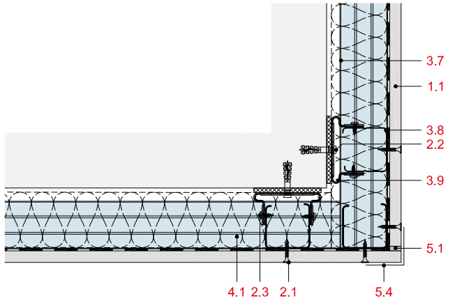
Ausbildung einer Außenecke, Vorsatzschale mit RigiProfil
