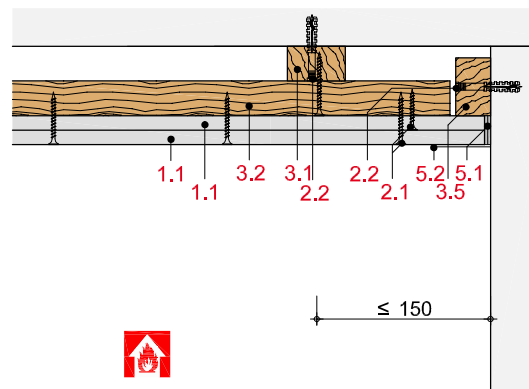
Schnitt B
