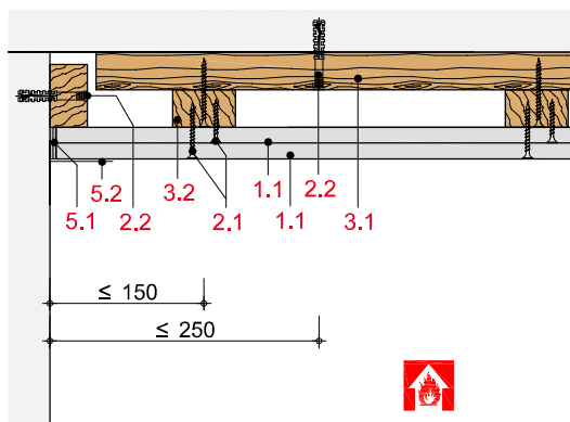
Schnitt A
