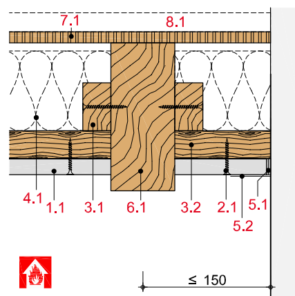
Schnitt B
