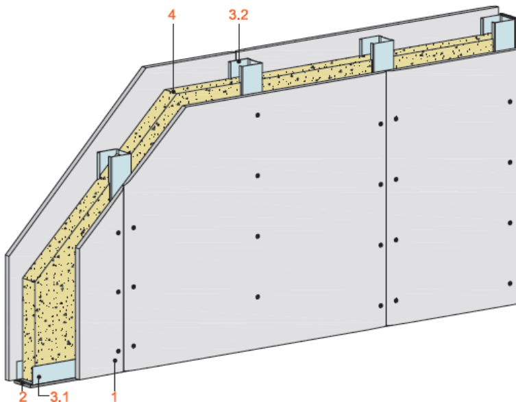
Abbildung 1: Trockenbausystem MW11RB/MW11RF/MW11DL
