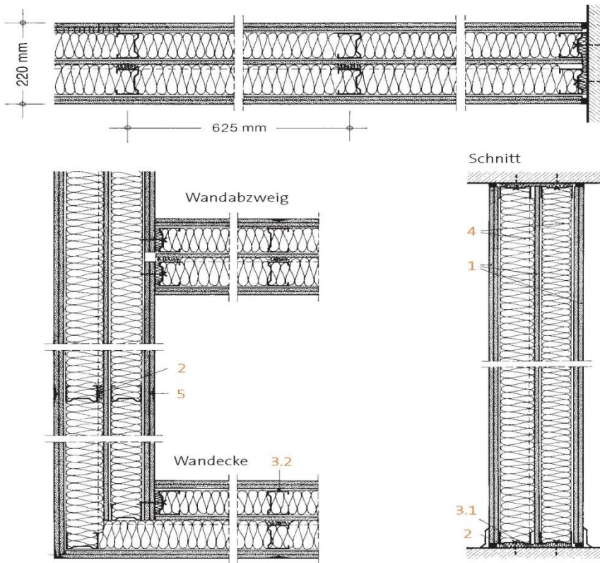
Abbildung 11: Trockenbausystem MW221RB/MW221RF
