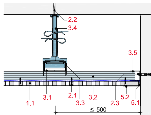
Schnitt B
