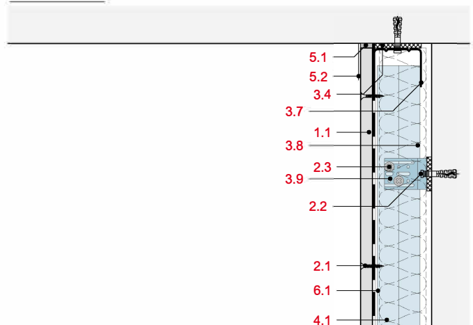
Deckenanschluss an Massivdecke, Vorsatzschale mit RigiProfil
