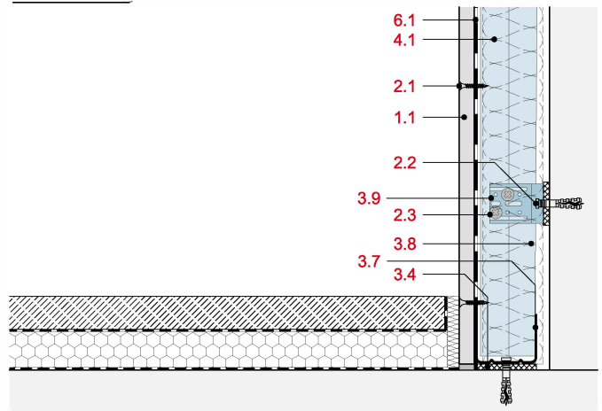
Bodenanschluss an Massivboden, Vorsatzschale mit RigiProfil
