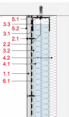
VS11-D-DM-1 Deckenanschluss an Massivdecke
