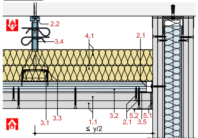
Längsschnitt
