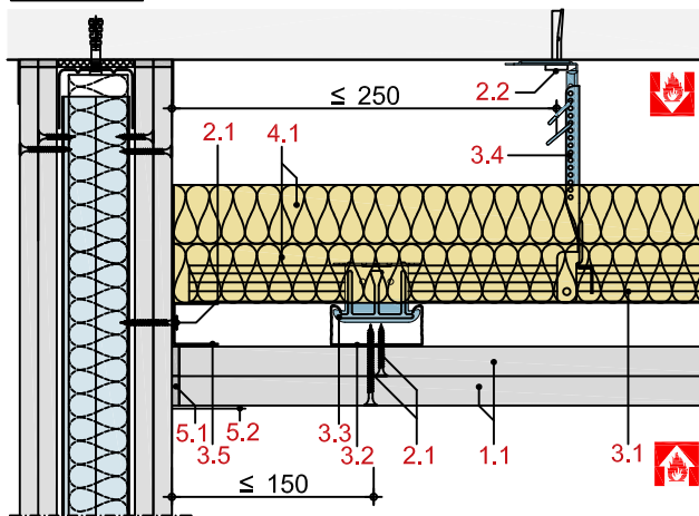
Querschnitt
