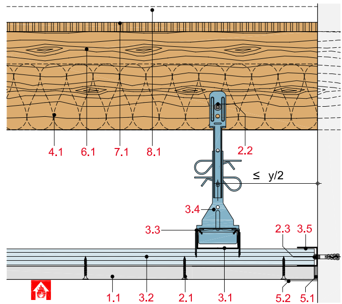
HB11 D WM30 2 Längsschnitt
