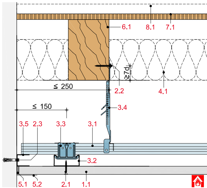
HB11 D WM30 1 Querschnitt
