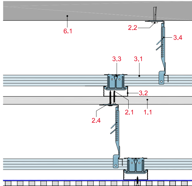
Rigips Sicht- bzw. Akustikdecke ( \leq 15 \text{ kg/m}^2 )
