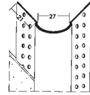
Außeneckprofil abgerundet* PVC-Kantenprofil weiß Länge 305 cm* für gebogene Kanten. Einsei- tig eingeschnittenes, abge- rundetes Kantenprofil aus PVC zur Herstellung von gebogenen GK-Konstrukti- onen. Profil von Hand biegen und vollflächig einspachteln.
