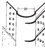
Außeneckprofil abgerundet* PVC-Kantenprofil Länge = 305 cm Einseitig eingeschnittenes, abgerundetes Kantenprofil aus PVC zur Herstellung von gebogenen GK- Konstruktionen. Profil von Hand biegen und voll- flächig einspachteln.
